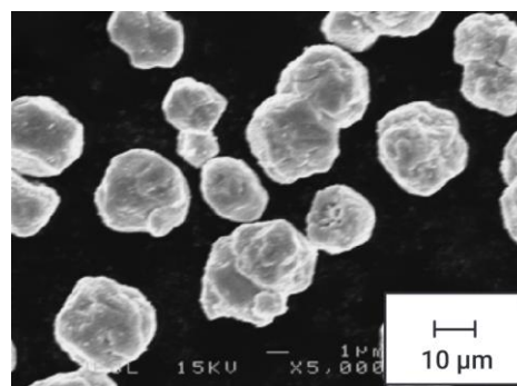
Электропроводящие частицы меди, покрытые серебром
